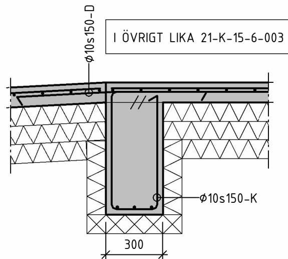
24 1 : 20 ANSLUTNING AV RAMP MOT SULA
