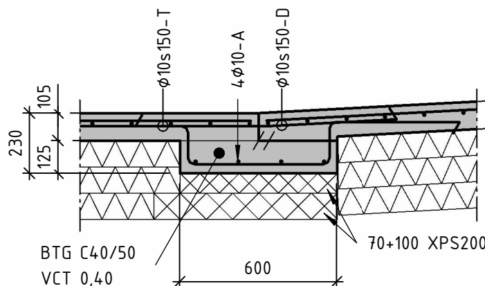
22 1 : 20 ANSLUTNING AV RAMP I BOTTEN
