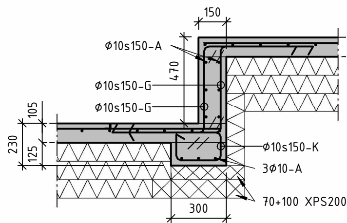
20 1 : 20 NIVÅSKILLNAD KAPPRUM
