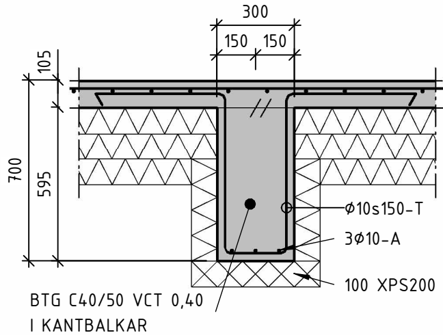
21 1 : 20 ANSLUTNING MOT SULA
