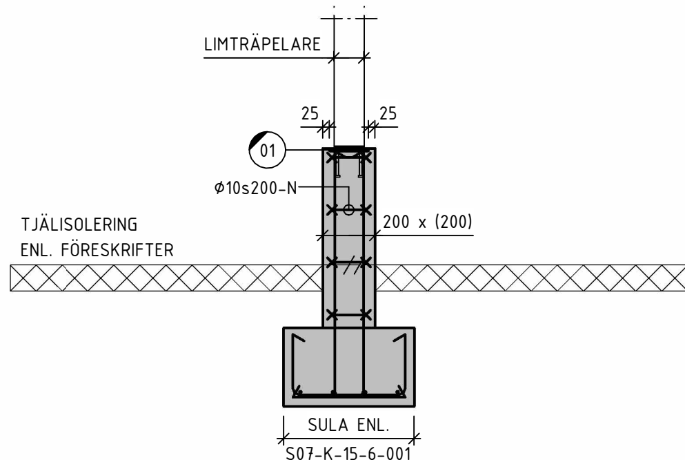
25 1 : 20 FUNDAMENT VID SKÄRMTAK VID ENTRÉ
