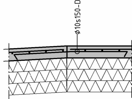
23 1 : 20 ANSLUTNING AV RAMP I TOPPEN
